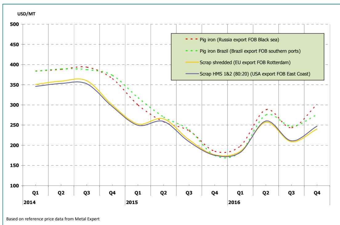
กราฟแสดงราคาวัตถุดิบอ้างอิงในตลาดโลก ช่วงไตรมาส 1/2557 – ไตรมาส 4/2559
