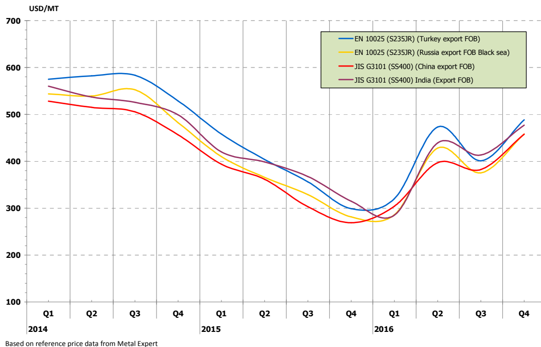
กราฟแสดงราคาเหล็กแผ่นรีดร้อนชนิดม้วนอ้างอิงในตลาดโลก ช่วงไตรมาส 1/2557 – ไตรมาส 4/2559
