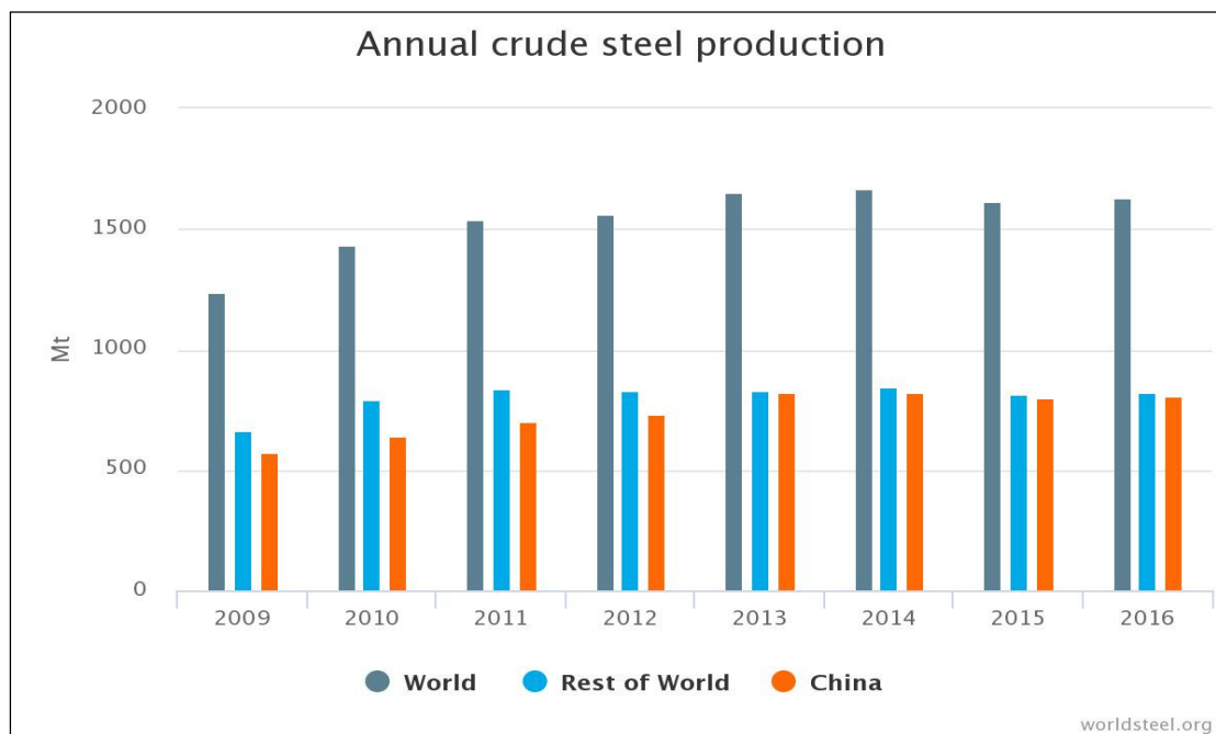
กราฟแสดงปริมาณการผลิตเหล็กดิบของโลก สิ้นสุด ณ 31 ธันวาคม 2559
